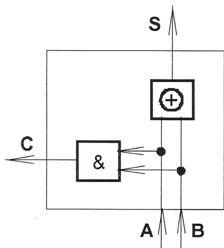
a.) félösszeadó
